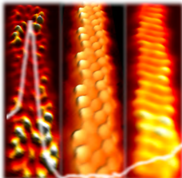
Figure 4: Descripción esquemática de la estructura electrónica de las nanotiras de grafeno de tipo quiral de anchura pequeña.
