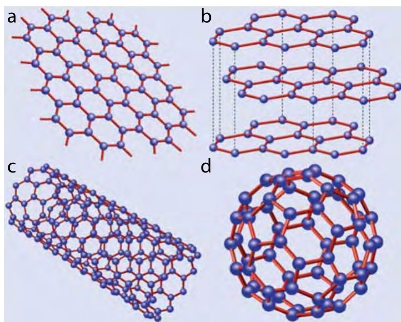
Figure 1: Modelos del grafeno y sus principales materiales derivados. (a) Grafeno, (b) grafito, (c) nanotubos, (d) fulerenos. Adaptado de ref. 8
